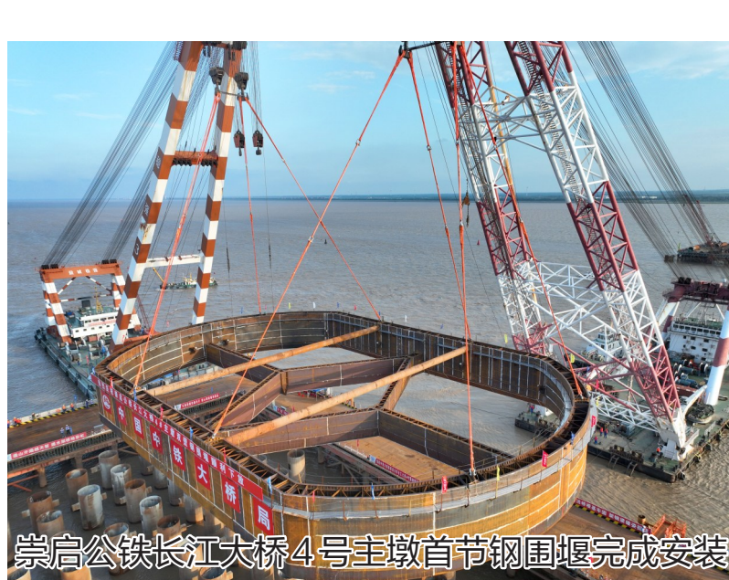
崇启公铁长江大桥4号主墩首节钢围堰完成安装
